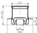
/13/ PVP 122x122 PR/DN 50 N
