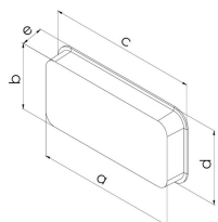
Műanyag csőlezáró idom / Plastikstopfen ZP 110x55
