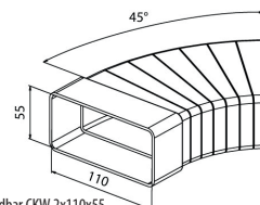
Állítható könyök idom (45°) / Flachkanal-Bogen, abschneidbar CKW 2x110x55
