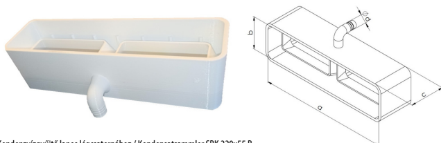
Kondenzvízgyűjtő lapos légszatórnához / Kondensatsammler SBK 220x55 B
